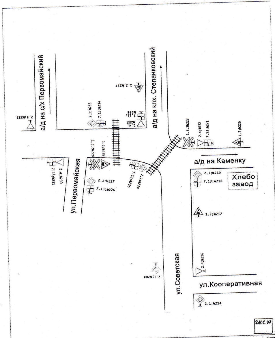
Схема размещения дорожных
